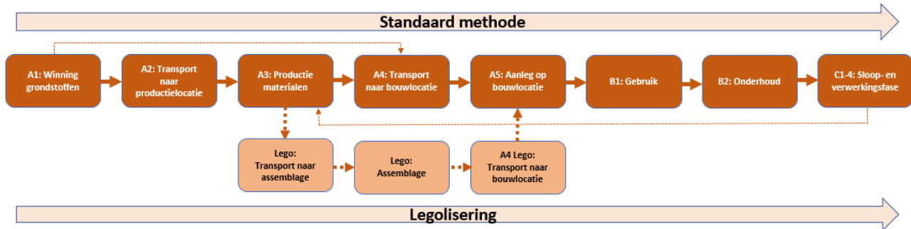
Figuur 1 Ketenmodel volgens de 'SBK Bepalingmethode Milieuprestatie Gebouwen en GWW werken'
