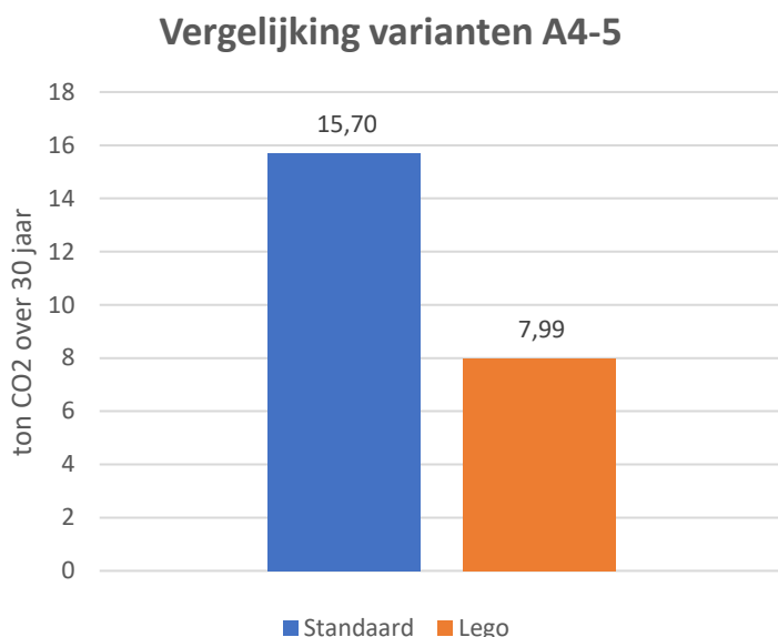
Figuur 4 Vergelijking varianten A4 en A5
